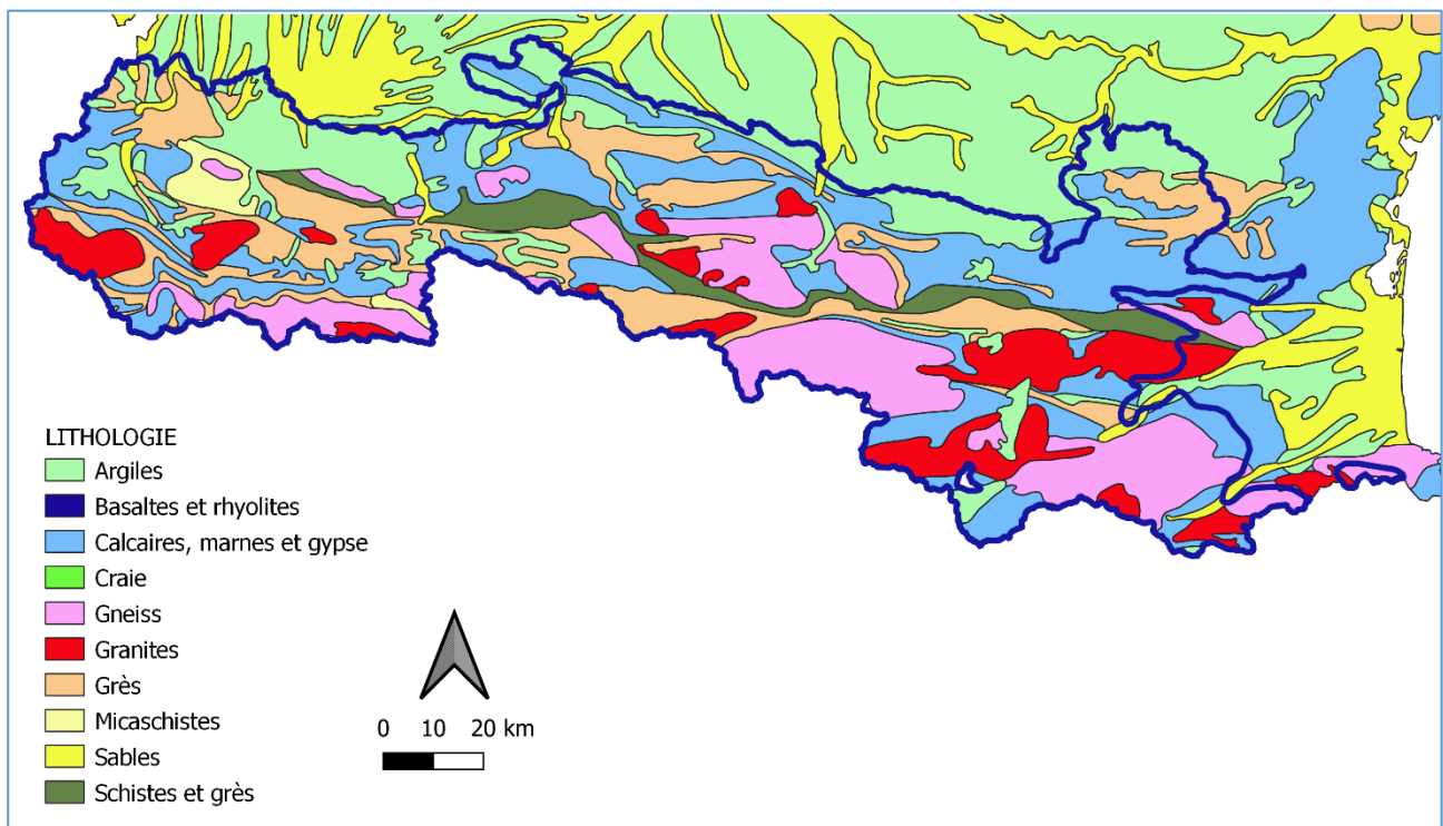
Carte 3 : Lithologie simplifiée des Pyrénées – Source BRGM
